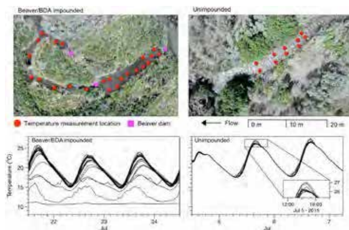
Abbildung 2: Links ein System mit Biberdämmen (pinkes Rechteck), rechts ein Gewässerabschnitt ohne Biberdämme. Beide Systeme zeigen ähnliche Höchsttemperaturen wobei im System ohne Biber keine große Temperaturvarianz zu erkennen ist. Die Temperaturvarianz im Bibergebiet zeigt, dass es lokal zur deutlichen Abkühlung kommt. (Quelle: https://journals.plos.org/plosone/article?id=10.1371/journal.pone.0176313 )
